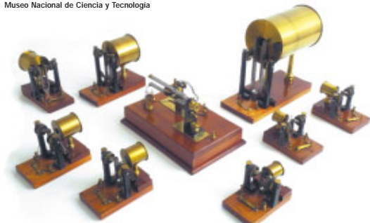
Sintetizador de Heilmholtz (1865 - 1890) Museo Nacional de Ciencia y Tecnología
